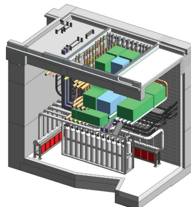
〈소화가스실 및 입상 배관 3D View〉
