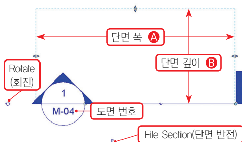
〈단면 기호〉
