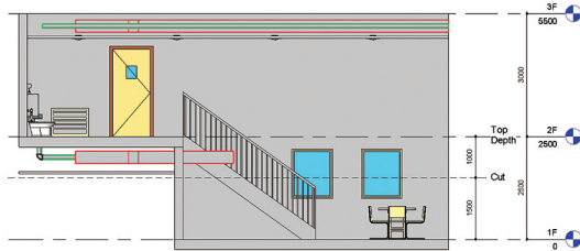
1F(Cut Plane을 1F에서 1500으로 설정)
