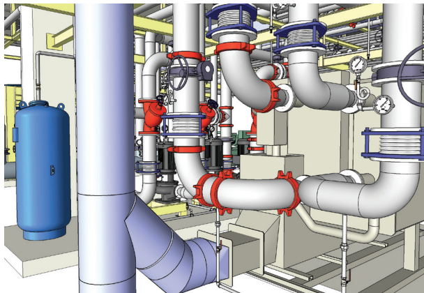
〈냉온수기 3D View〉
