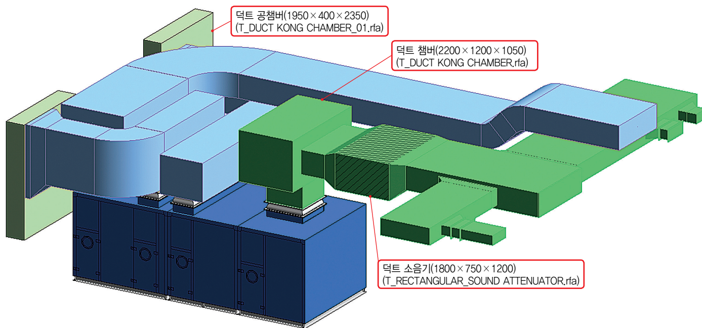
〈공조실 3D 뷰〉
