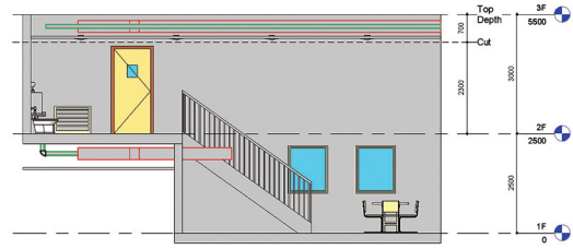
2F(Cut Plane을 2F에서 2300으로 설정)
