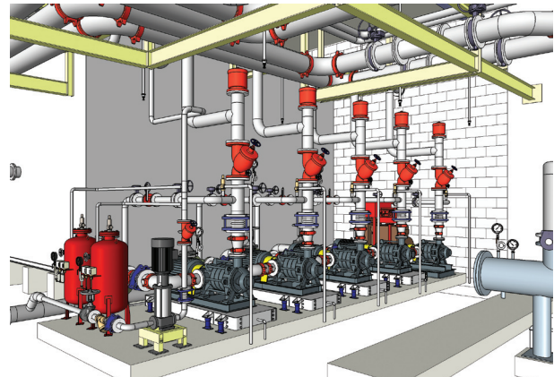
〈소방 펌프 3D View〉
