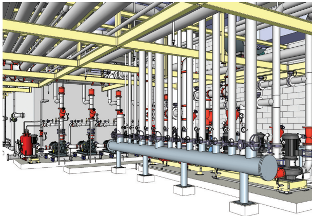
〈냉온수 헤더 3D View〉
