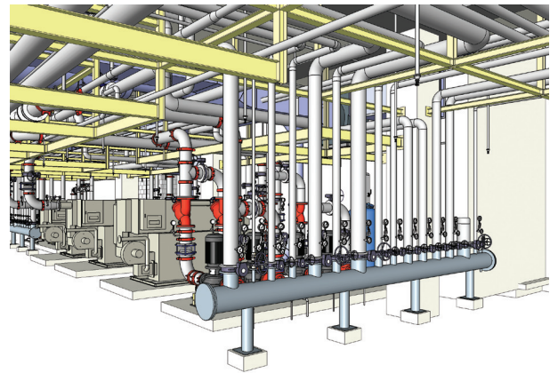
〈냉온수 헤더 3D View〉
